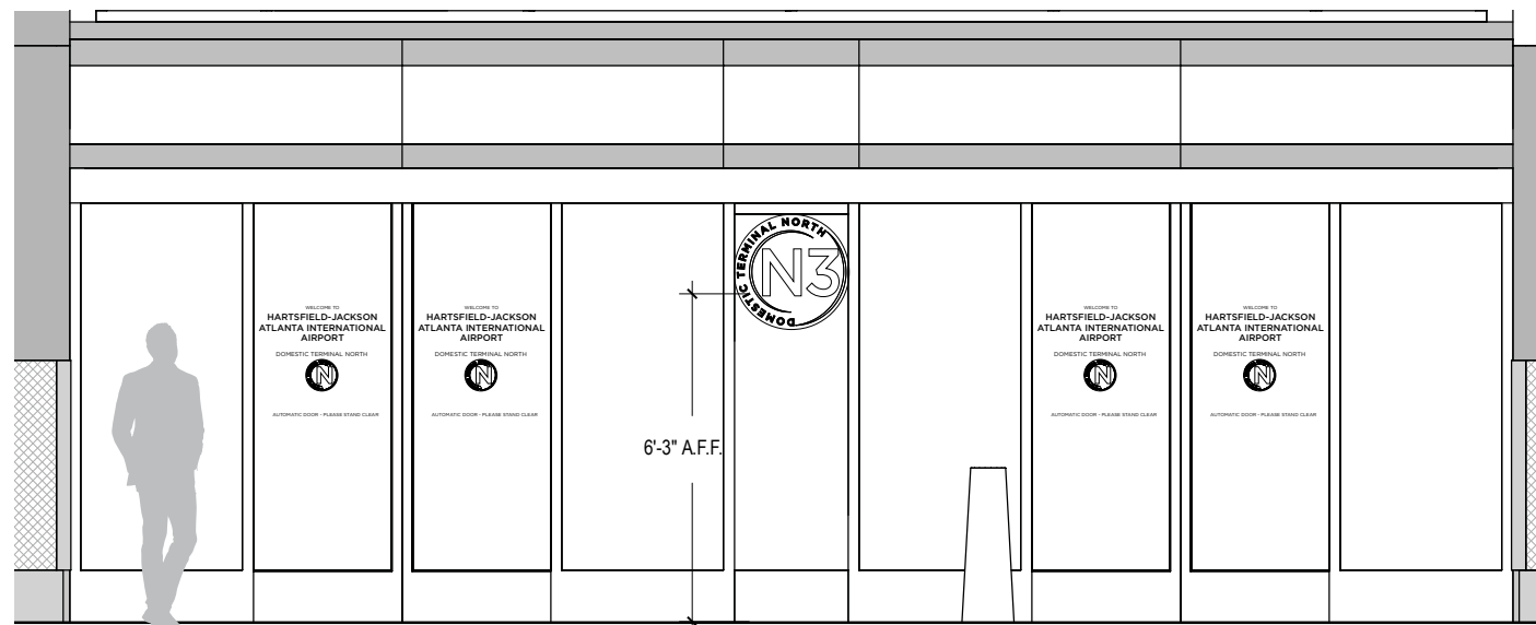
2 ELEVATION SCALE: 1/4" = 1' - 0"
