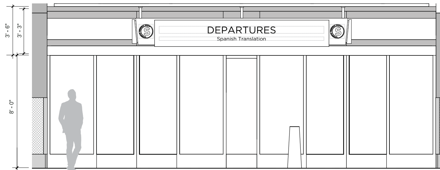
4 ELEVATION SCALE: 1/4" = 1' - 0"
