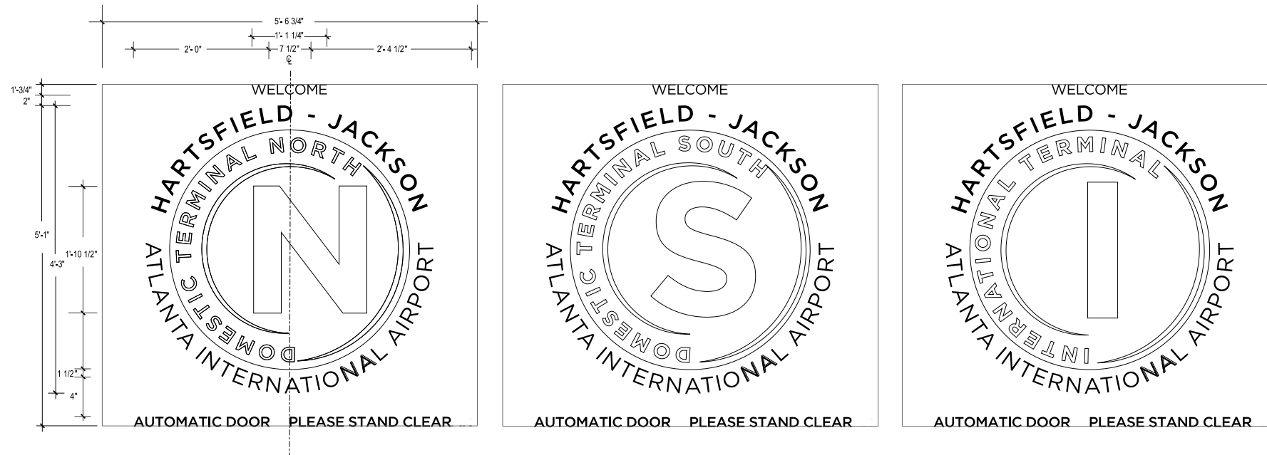
1 TERMINAL IDENTIFICATION SCALE: 3" = 1' - 0"
