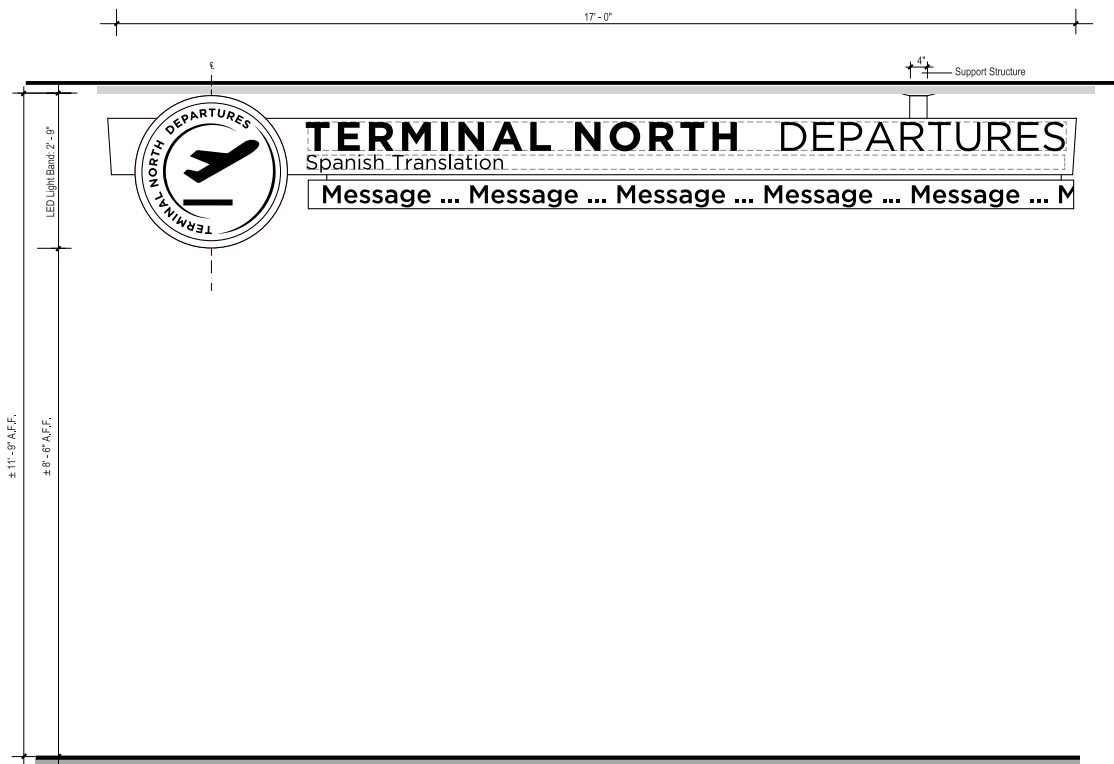
7 ELEVATION SCALE: 1/2" = 1' - 0"
