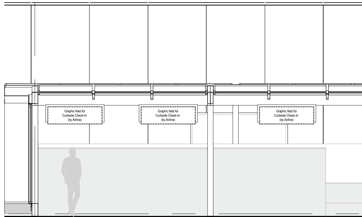
4 ELEVATION SCALE: 1/4" = 1' - 0"
