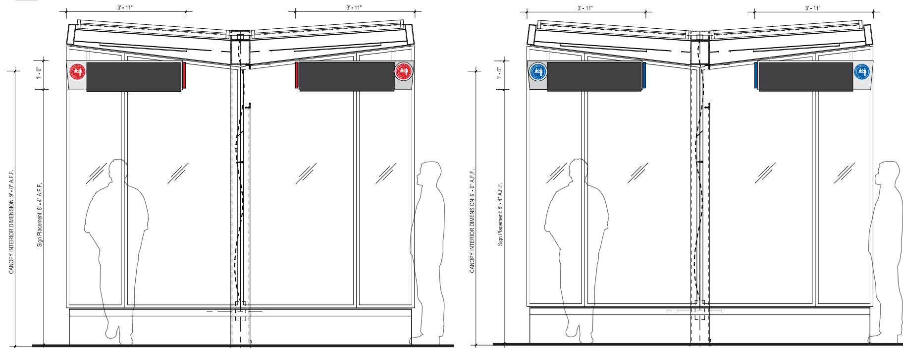
5 ELEVATION SCALE: 1/2" = 1'-0"
