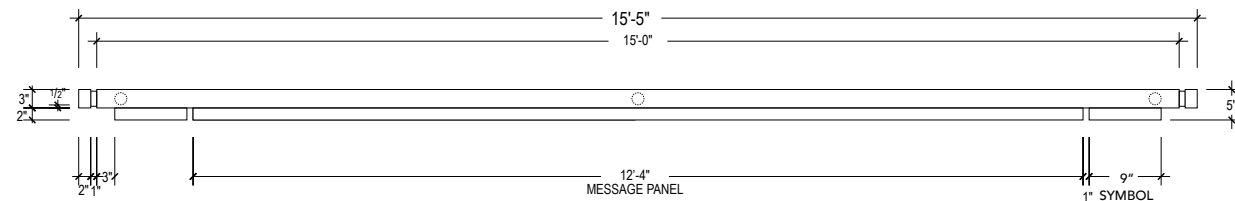
1 TOP VIEW SCALE: 1/2" = 1' - 0"
