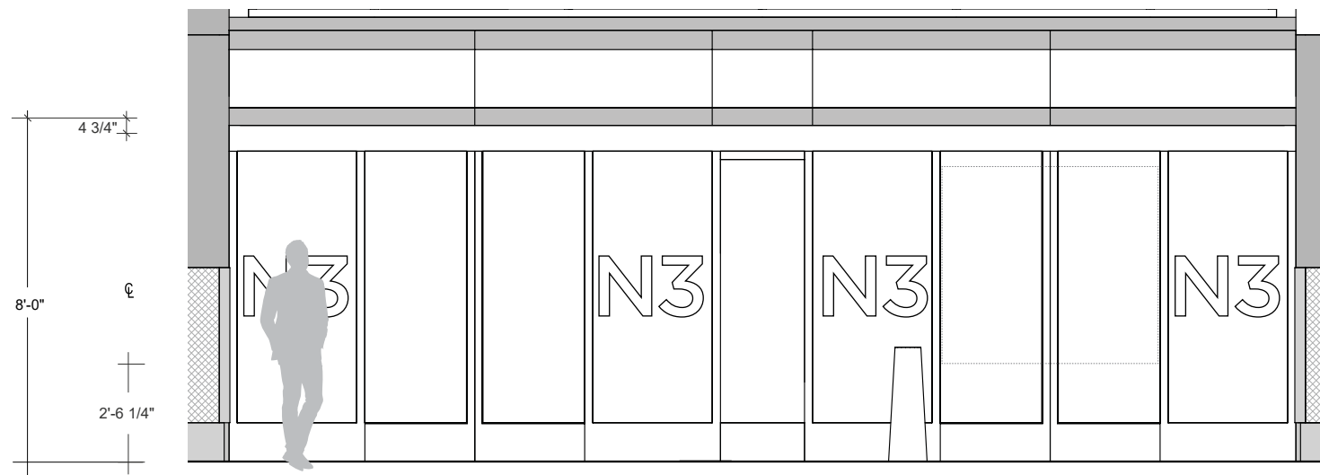
2 ELEVATION SCALE: 1/4" = 1' - 0"
