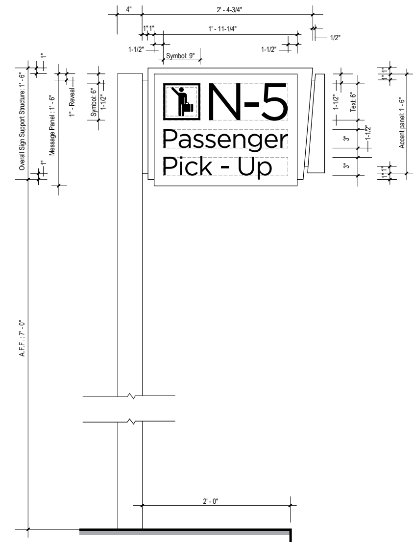
4 ELEVATION SCALE: 1" = 1' - 0"
