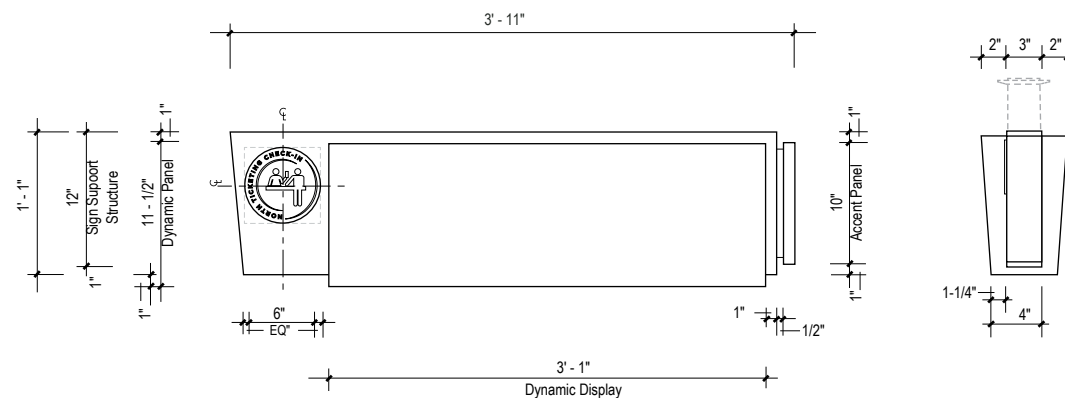
7 FRONT VIEW SCALE: 1" = 1'-0"
