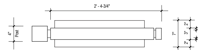
5 TOP VIEW SCALE: 1" = 1' - 0"
