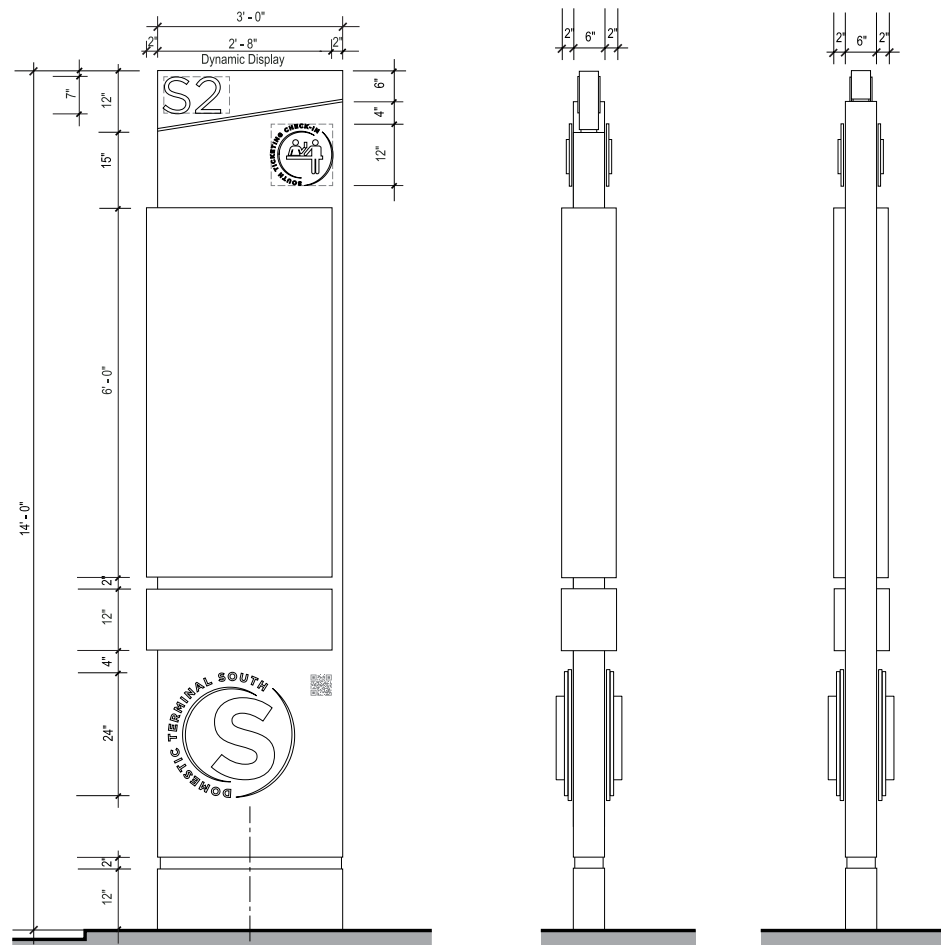
9 FACE LAYOUT SCALE: NTS
